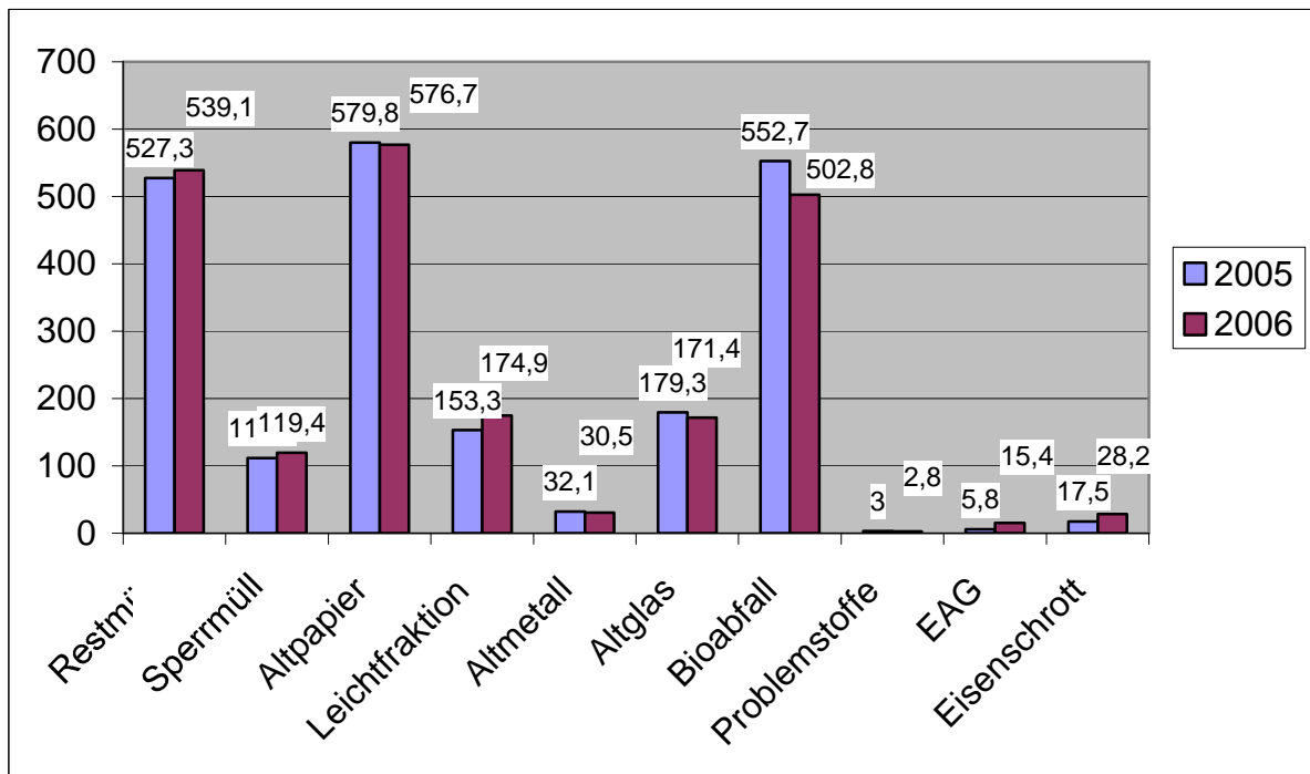
Diagramm 3: Gesamtmengenvergleich 2005 - 2006
